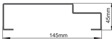
Detalle de Marco Chapa #18
